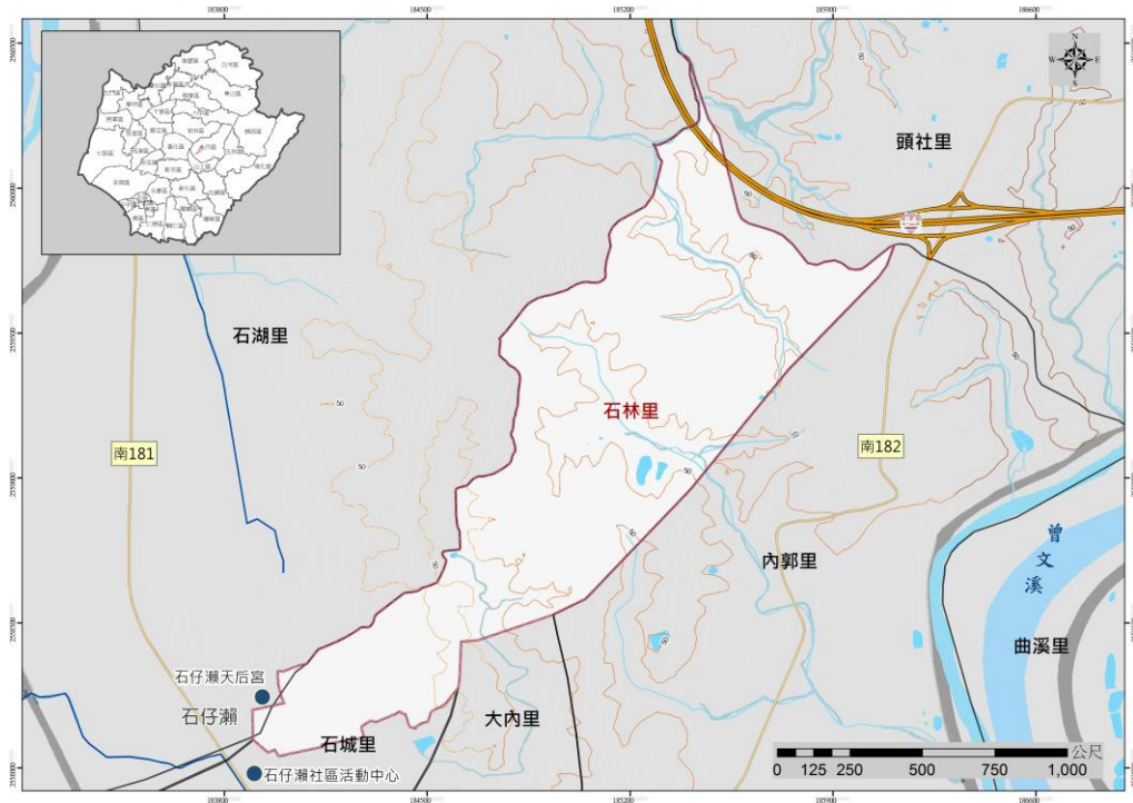
圖 1 臺南市大內區石林里地理位置圖
